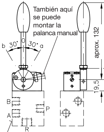
Superficie de brida en válvula de corredera SP 1
