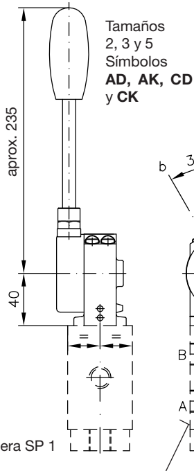
Superficie de brida en válvula de corredera SP 3(5)
